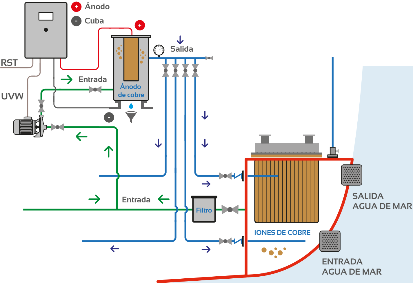
Esquema de conexión ELECTROPACK con BOXCOOLER
