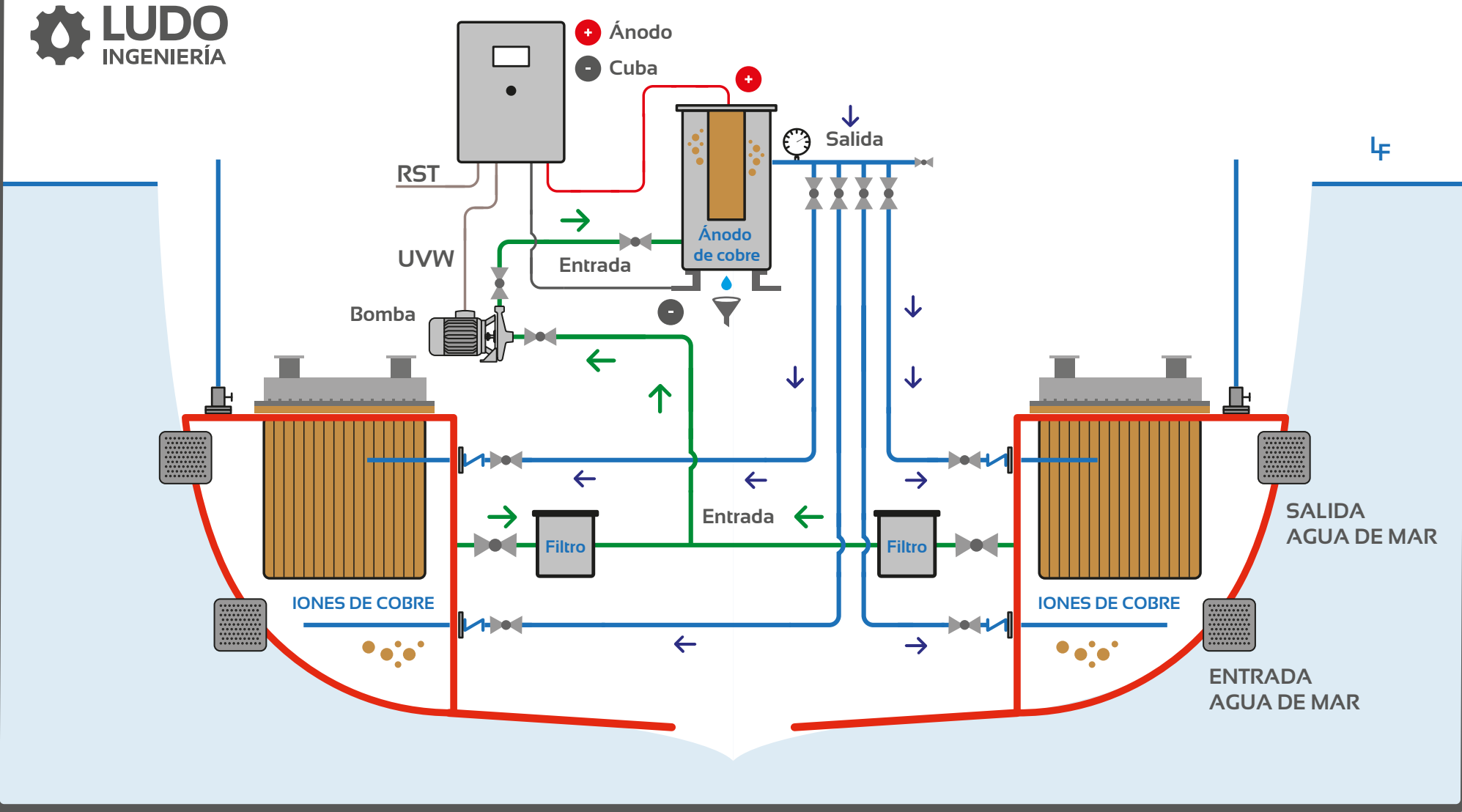
Esquema de conexión ELECTROPACK con BOXCOOLER
